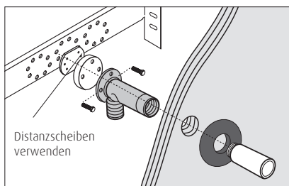
Doppelte Beplankung
