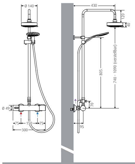
WimTec ECOSAN S6 KB mit Kopfbrause/Handbrause-Set (Art.Nr. 128 611)
