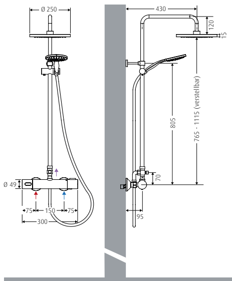
WimTec ECOSAN S6 KB mit Regendusche/Handbrause-Set (Art.Nr. 128 604)
