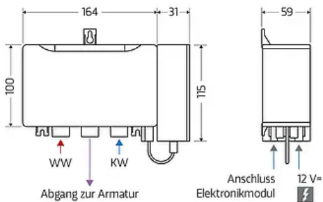
Elektronischer Thermostat
