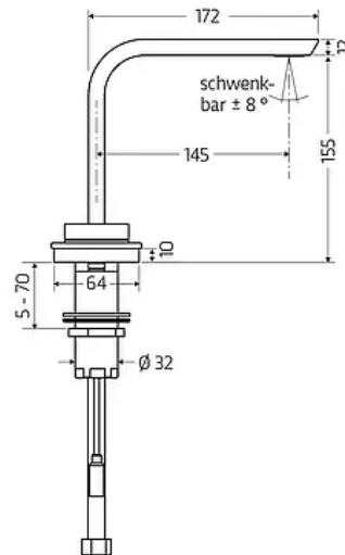
Montage
