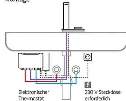
Montage
