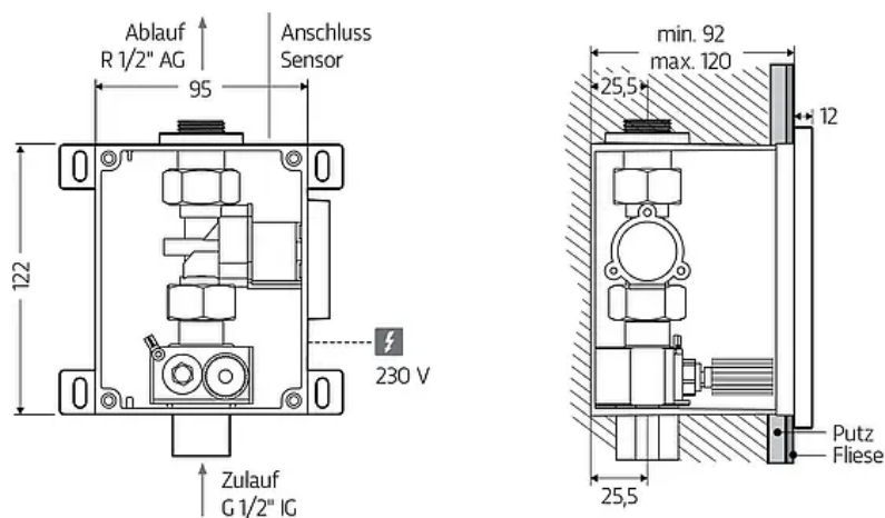
Produkt: Maße in mm
