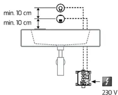
Montage: Maße in cm
