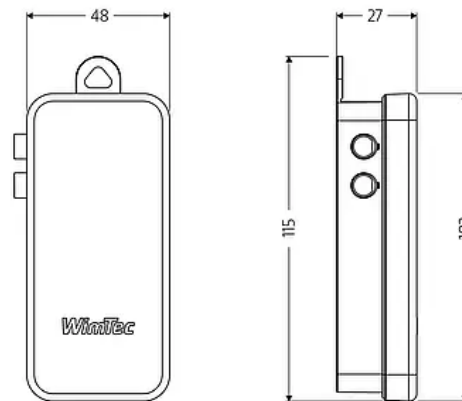
WimTec PROOF SV - Elektronikmodul:
