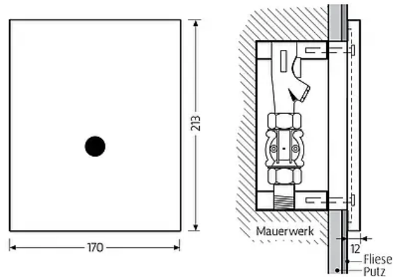
Produkt: Maße in mm
