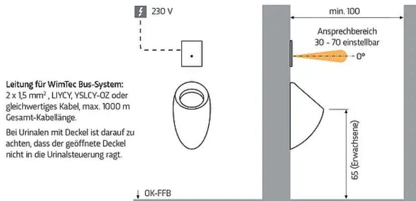
Montage: Maße in cm
