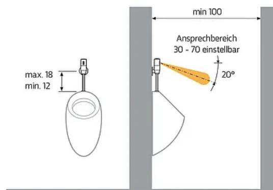
Montage: Maße in cm
