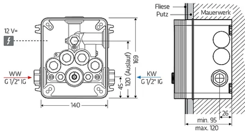
Montage: Maße in cm
