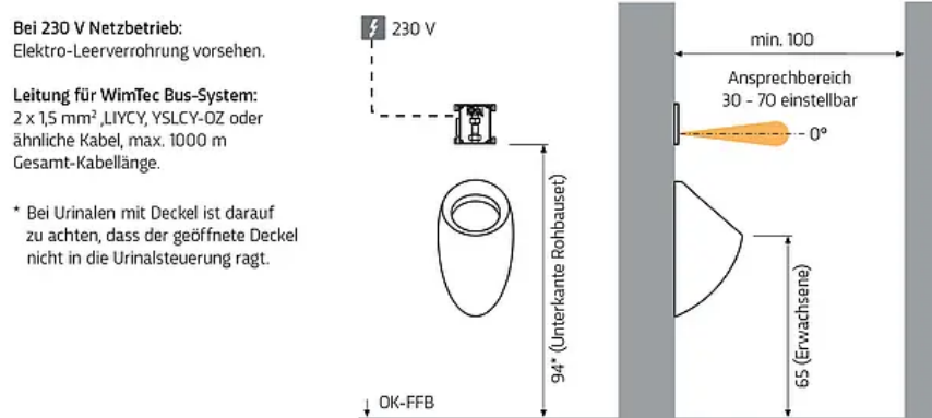
Montage: Maße in cm
