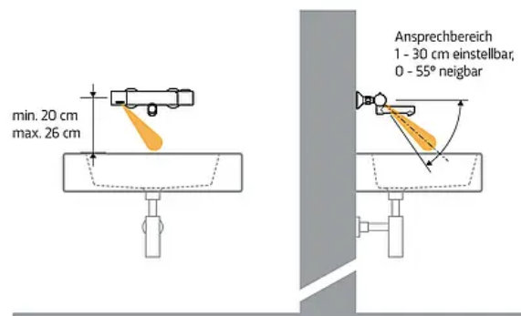
Montage: Maße in mm
