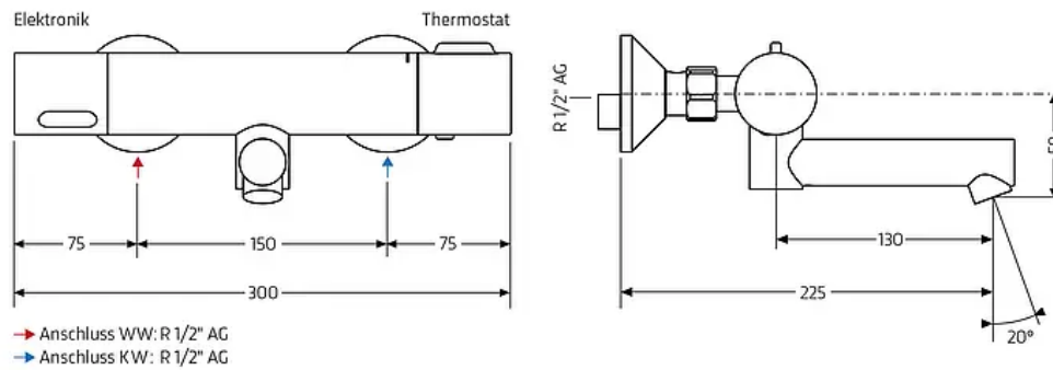
Produkt: Maße in mm
